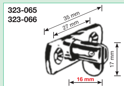
323-065 Fissaggio orizzontale doppio telo bianco Horizontal fixing double fabric, white color 323-066 Fissaggio orizzontale doppio telo nero Horizontal fixing double fabric, black color
