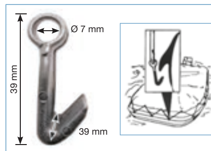
20280 Gancetto per gommoni (20pz) col. bianco/grigio/nero Nylon hook for dinghies (20pcs) col. white/grey/black
