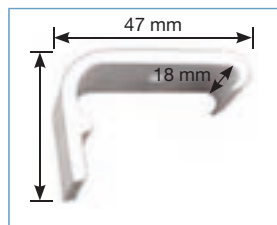
20008 Fermo per capottine col. Bianco/nero Fastener for capote col. White/black
