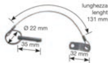
207-000 Piastrina inox + cavetto inox Ø 1.6mm + spina inox con bloccaggio a sferetta
