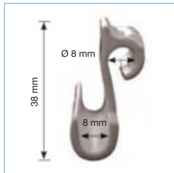
20031 Gancio per corda elastica aperto col. bianco/*nero/*grigio Hook for elastic cord col. white/*black/*grey
