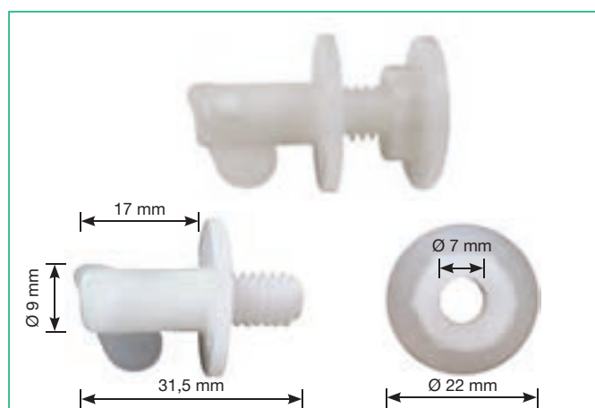
323-055 Fissaggio telo-telo doppio tessuto bianco Canvas to canvas double, white color 323-053 Fissaggio telo-telo doppio tessuto nero Canvas to canvas double, black color
