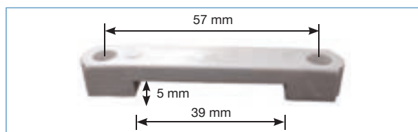
20033 Fissaggio per 20031 e 20032 col. bianco/*nero/*grigio Fastener for 20031 and 20032 col. white/*black/*grey
