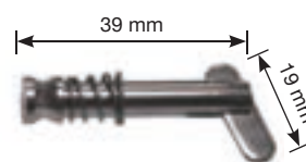
207-002 Spinetta cavalletto reggi cappottina Ø 6mm in inox
