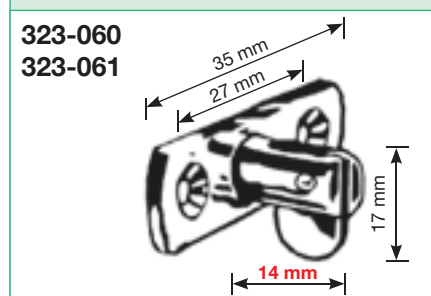
323-060 Fissaggio orizzontale bianco Horizontal fixing, white color 323-061 Fissaggio orizzontale nero Horizontal fixing, black color
